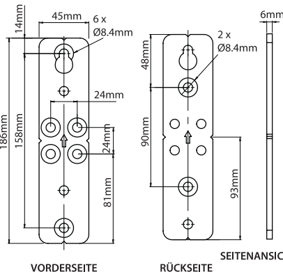
VORDERSEITE
