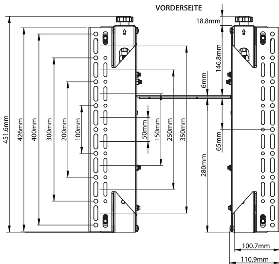
VORDERSEITE
