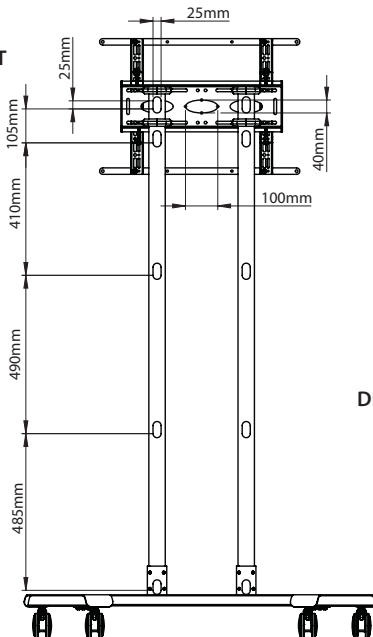
RÜCKANSICHT
