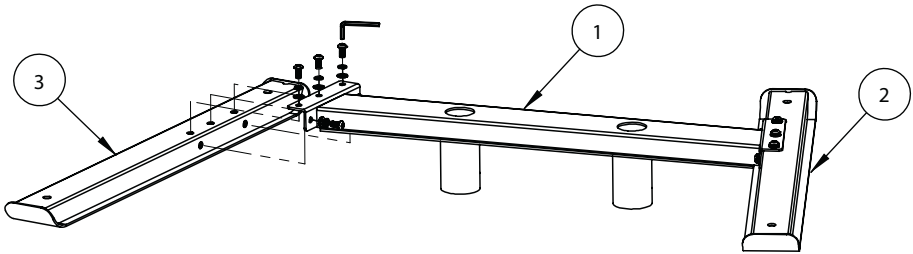
M8 x 16mm SCHRAUBE
