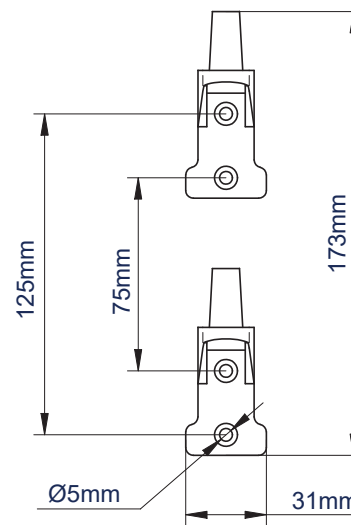
WALL HINGES
