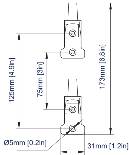
WALL HINGES
