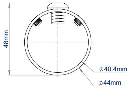
DRAUFSICHT
