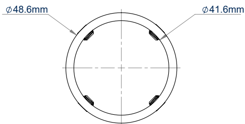
BOVENAANZICHT
