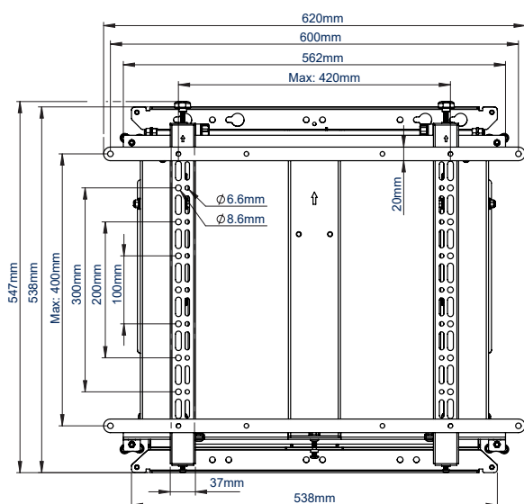
VOORAANZICHT MET ADAPTERARMEN
