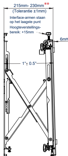
ZIJ AANZICHT OPEN
