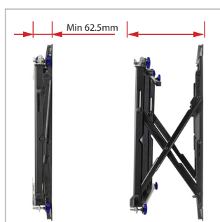
Het slimline design met gedempte opening zorgt voor een snelle toegang tot de achterkant van de schermen
