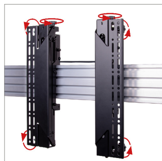
Werkzeuglose Fein-Justage für nahtlose Display-Ausrichtung
