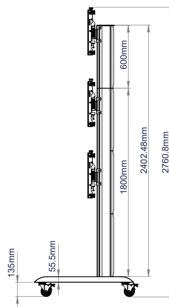
SEITENANSICHT
