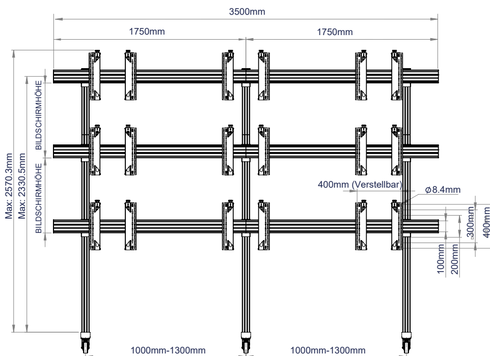
VORDERANSICHT
