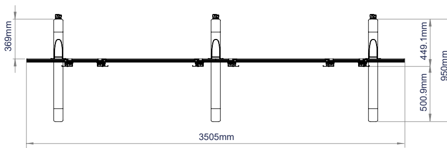
DRAUFSICHT
