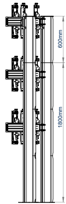
SEITENANSICHT
