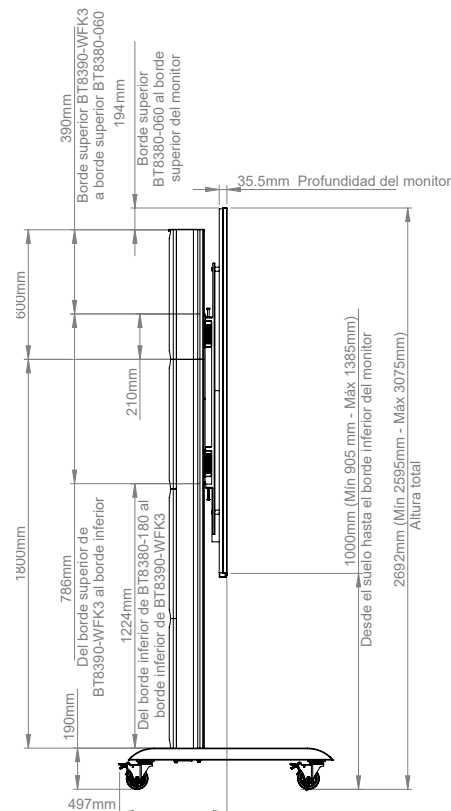
DETALLE A ESCALA 1 : 5
