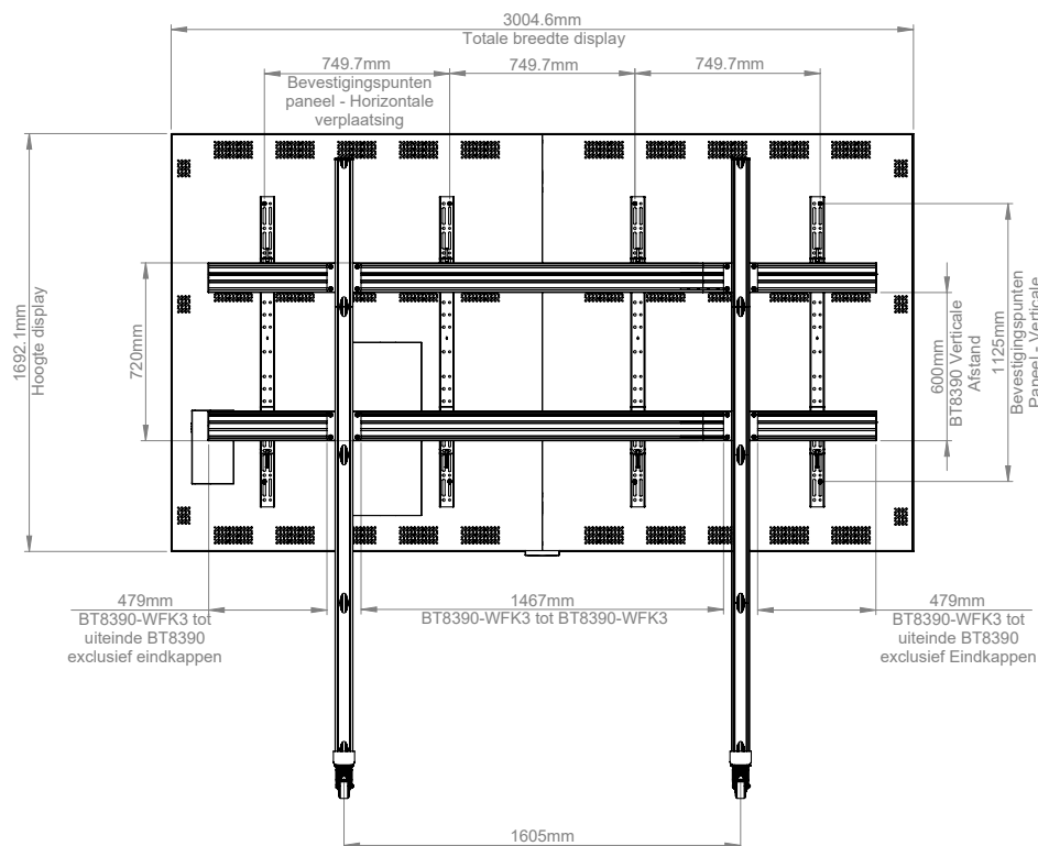
ACHTERAANZICHT
