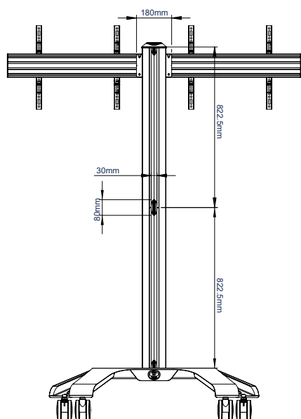
ACHTERAANZICHT
