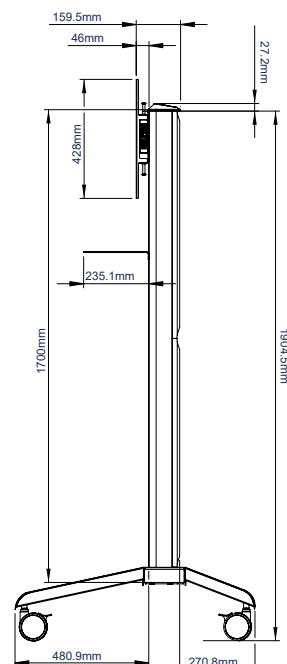
ZIJ AANZICHT
