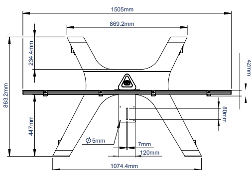
BOVENAANZICHT
