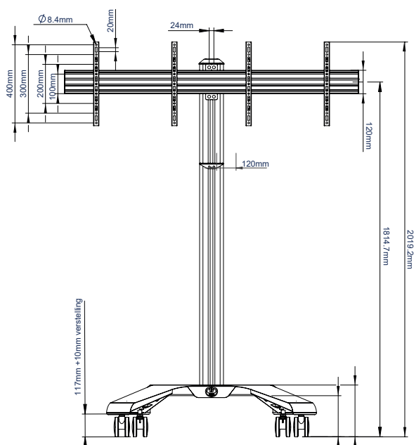
VOORAANZICHT
