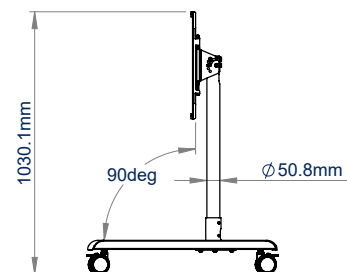
90° TILT
