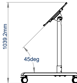
45° TILT
