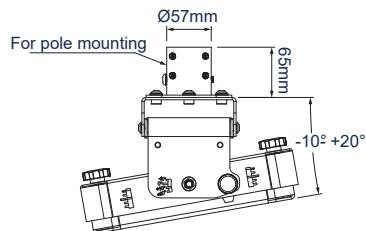
WIDOK Z BOKU Z ADAPTEREM WYSIEGNIKA
