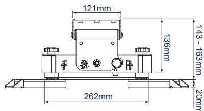
WIDOK Z BOKU Z KRÓTSZYMI RAMIONAMI
