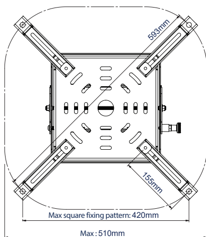
WIDOK Z DOŁU Z KRÓTSZYMI RAMIONAMI
