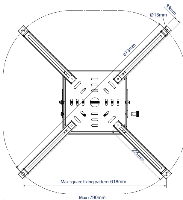
WIDOK Z DOŁU Z DŁUŻSZYMI RAMIONAMI
